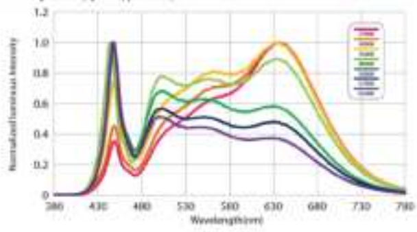
Color Spectrum ( T_1=25^{\circ}\text{C} , I_f=450\text{mA} )
